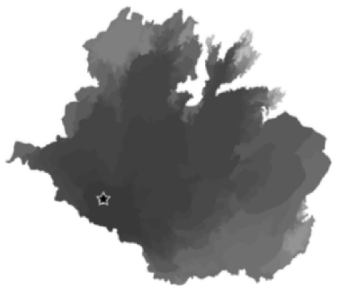
e) Reversed YIOrrd
