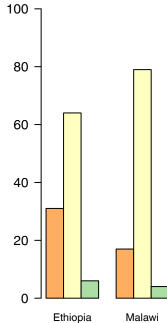
(d) Poster 4a (Raw probability)
